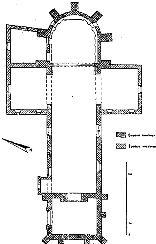
Saint-Martin de Légnacq. Plan d'ensemble
